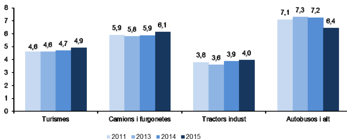
Gràfic 6 Pes del parc de vehicles del Bages sobre Catalunya. 2011-2015 Dades en %
